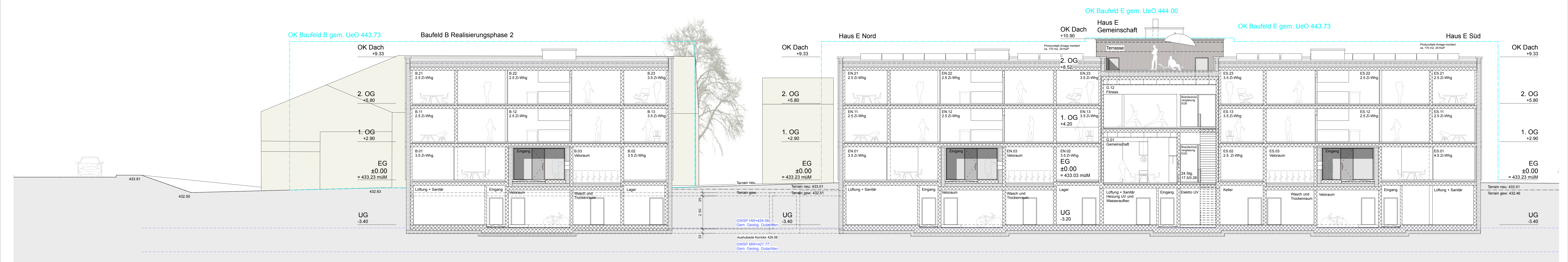
Schnitt C-C Längsschnitt M 1:100 Parzelle 299/1175
